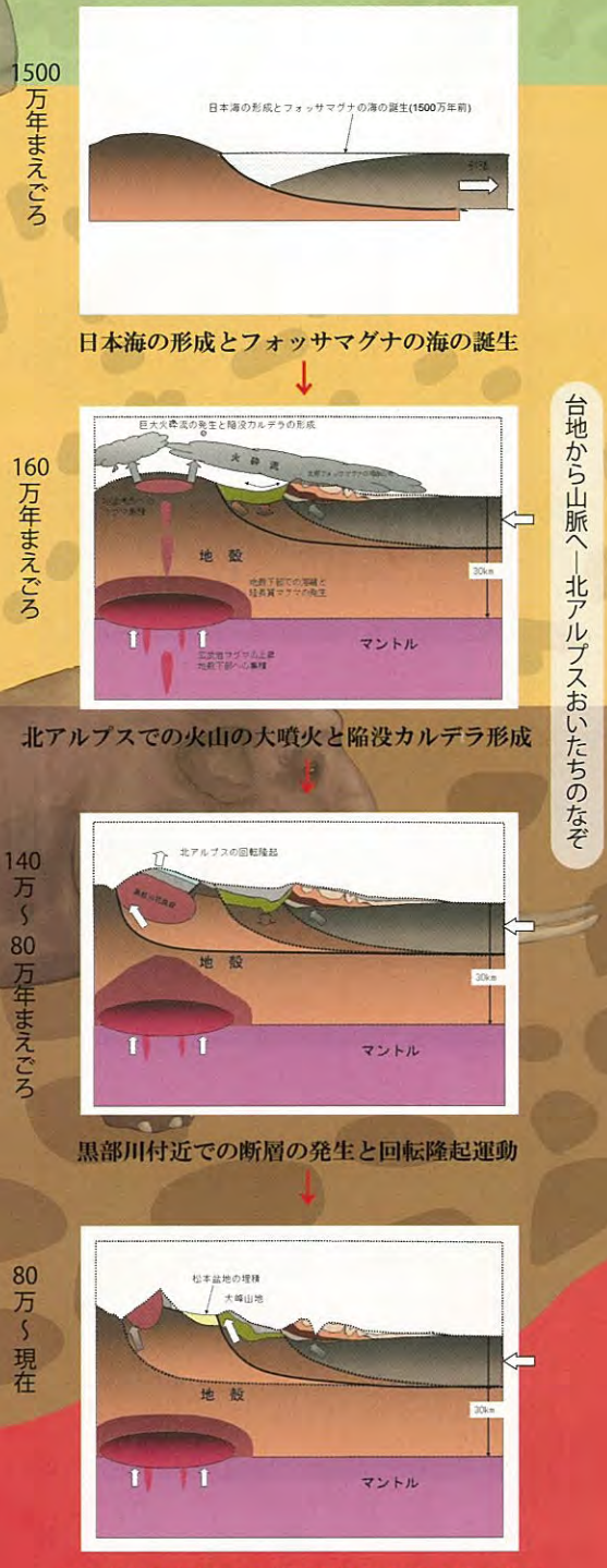
松本盆地東縁断層の活動開始と大峰山地の隆起
